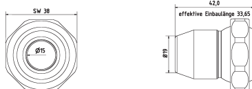
Boquilla de salida de Ø15 mm
