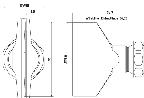
3-DU-SL-76-GS-1.0
