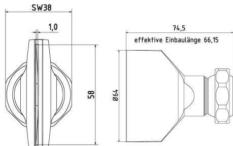
3-DU-SL-65-GS-1.0
