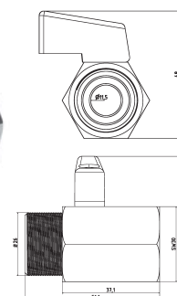
Mini-válvula de bola G 3/4" Latón cromado
