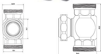
Pieza en T desplazable
