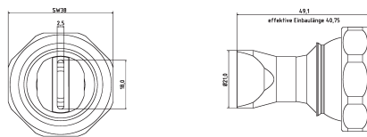
Boquilla de salida de 18 x 2,5 mm Chorro recto
