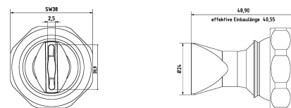
Boquilla de salida de 20 x 2,5 mm Chorro disperso
