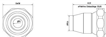
Boquilla de salida de Ø12 mm
