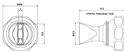
Boquilla de salida de 22 x 4,0 mm Chorro disperso
