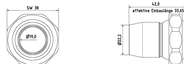
Boquilla de salida de Ø19 mm
