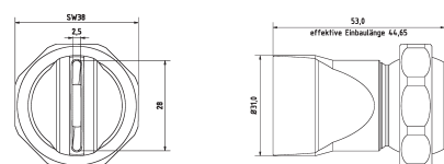
Boquilla de salida de 28 x 2,5 mm Chorro recto
