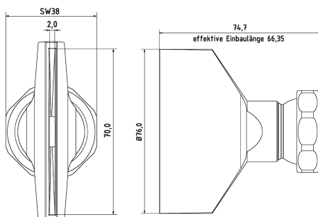
3-DU-SL-76-GS
