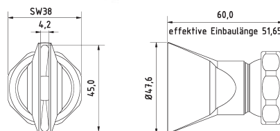
Boquilla de salida de 45 x 4,2 mm Chorro disperso
