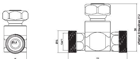
1-WV-2K Salida en T regulable
