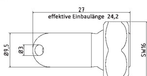
1-DU-30 Boquilla 30° de Ø3 mm
