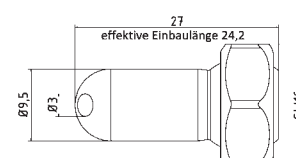
1-DU-60 Boquilla 60° de Ø3 mm
