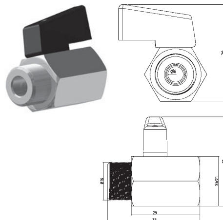
Válvula de 1/4 acero inoxidable
