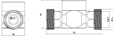
1-WV-2 Salida en T fija
