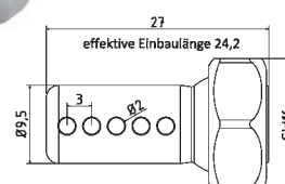
1-DU-90-5 Boquilla 90° de 5xØ2 mm
