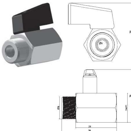
Válvula de 1/4 de Latón cromado
