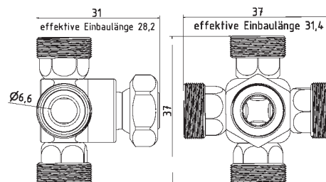
1-WV-4K Salida en Estrella regulable
