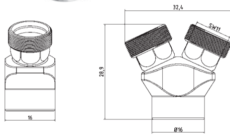
1-YV Salida en Y 50°
