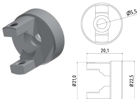
Soporte para salida (incluido tornillo)
