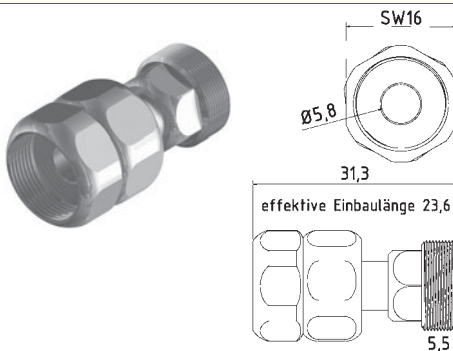
Elemento intermedio con posición fija (acoplamiento rápido)
