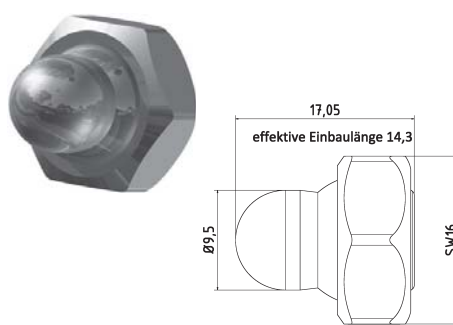
Tapon para salidas
