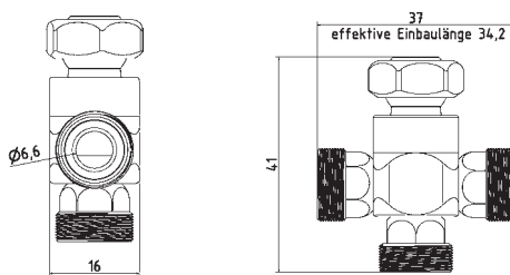
1-WV-3K Salida en Cruz regulable
