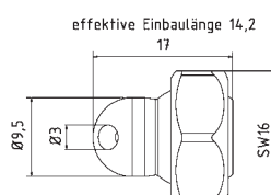
1-DU-30-EK Boquilla 30° de Ø3 mm extra corta
